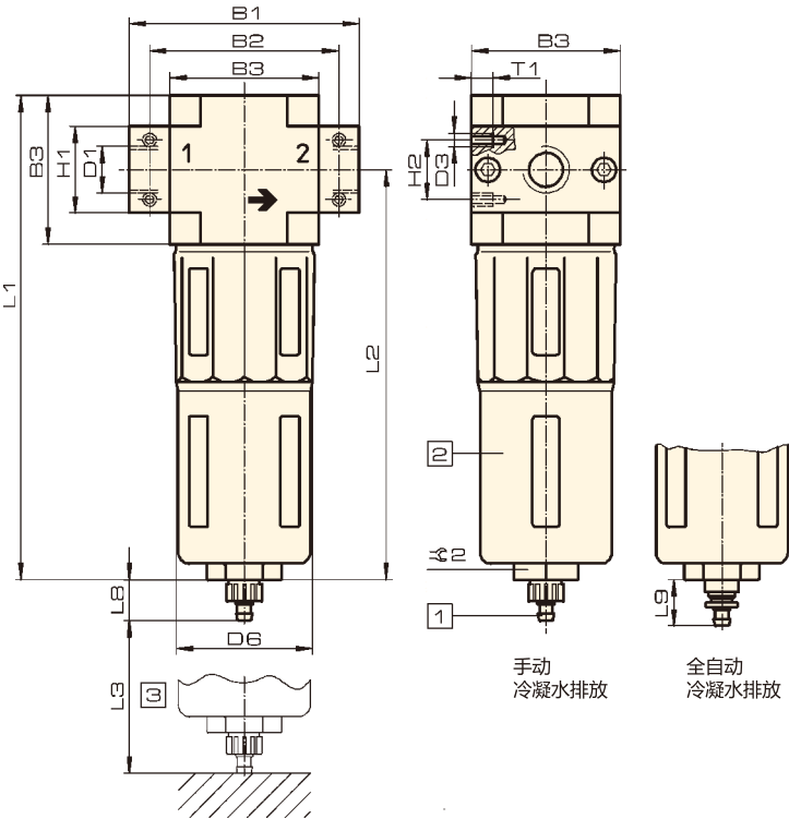
1 倒钩接头，用于塑料气管PCN-4 2 金属保护罩 3 安装尺寸 → 气流方向
